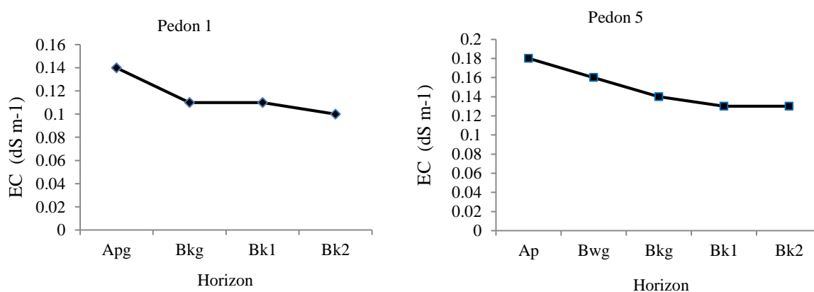
شکل ۵- تغییرات EC در افق‌های مختلف، دو خاکرخ مورد مطالعه
