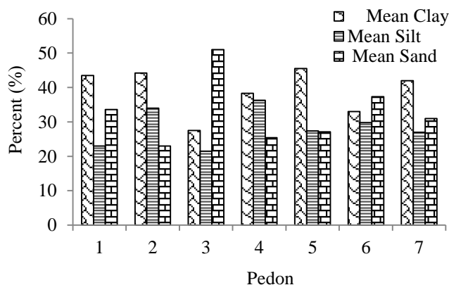
شکل ۴- مقایسه میانگین درصد توزیع ذرات، خاکرخ‌های مورد مطالعه
