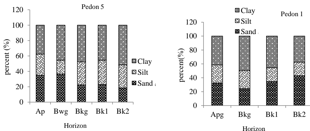
شکل ۳- توزیع اندازه ذرات در دو خاکرخ مورد مطالعه
