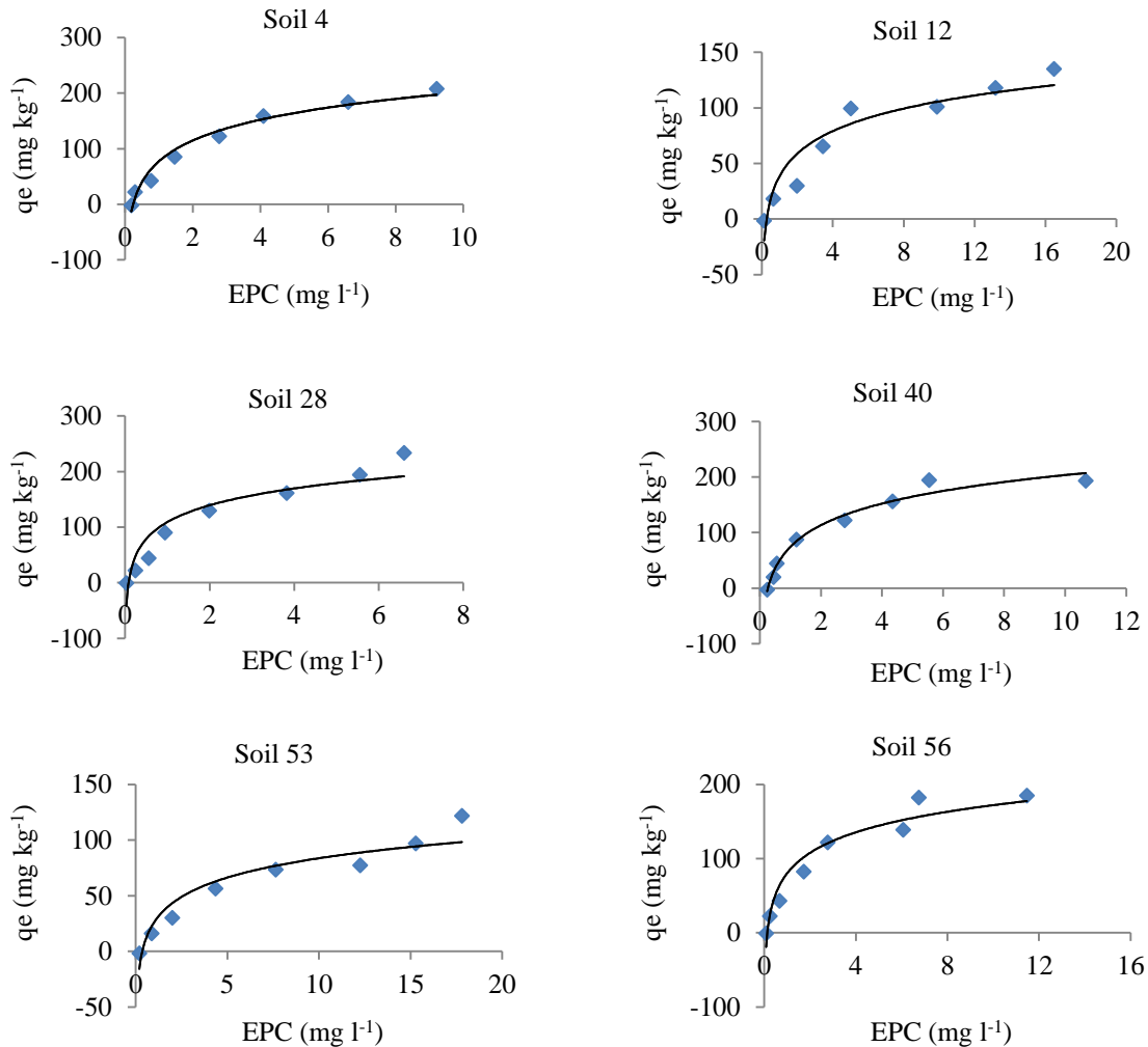
شکل ۲- روند جذب فسفر در برخی از خاک های مورد مطالعه Figure 2. Phosphorus sorption behaviour in some studied soils
