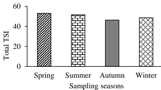
شکل ۸- تغییرات TSI کل تالاب کانی برازان در فصول مختلف
