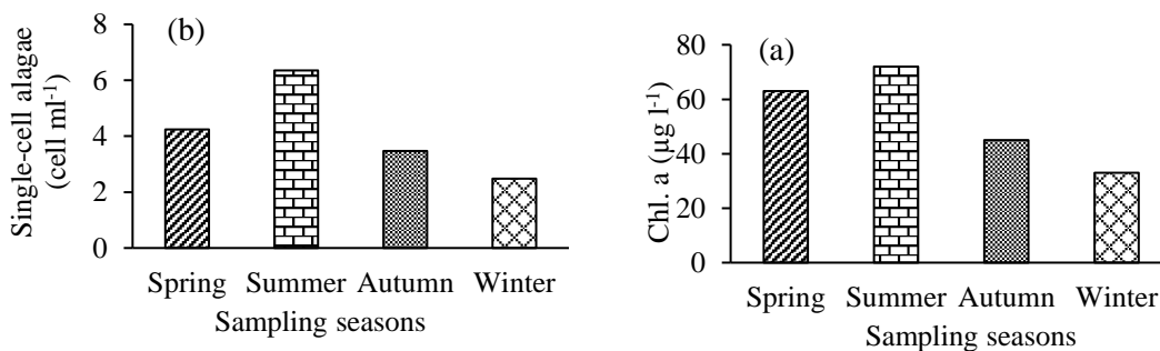
شکل ۷- مقایسه روند تغییرات TSI (Chl. a) و تراکم جلبک‌های تک سلولی در تالاب کانی برازان در فصول مختلف
