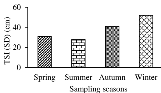
شکل ۶- روند تغییرات TSI (SD) در تالاب کانی برازان در فصول مختلف
