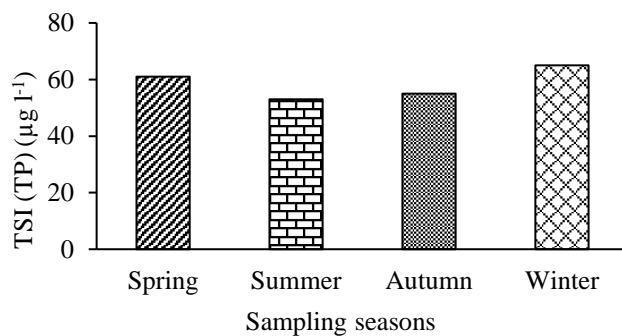
شکل ۵- روند تغییرات TSI (TP) در تالاب کانی برازان در فصول مختلف
