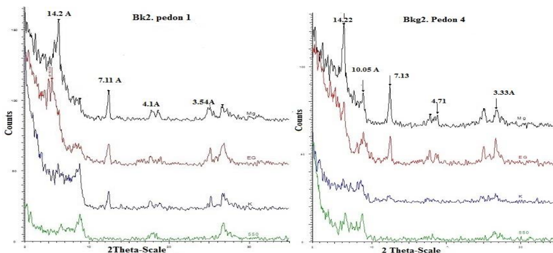
شکل ۸- دو نمونه از منحنی‌های پراش پرتو ایکس
