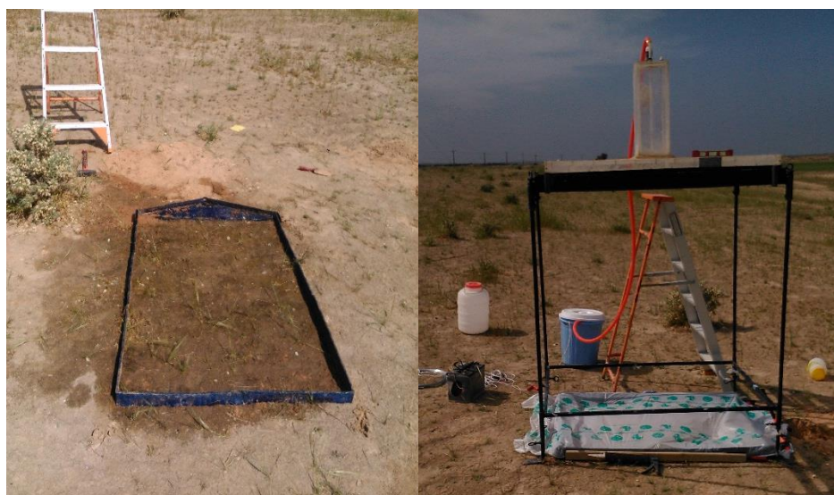
شکل ۲- سامانه شبیه‌ساز باران و تجهیزات آن
