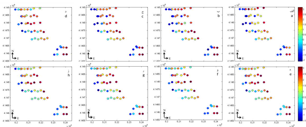
شکل ۲- موقعیت و مقادیر اندازه‌گیری شده EC خاک در بازه‌های زمانی مختلف. الف) بهار ۱۳۸۹؛ ب) پائیز ۱۳۸۹؛ ج) پائیز ۱۳۹۰؛ د) پائیز ۱۳۹۳؛ ه) بهار ۱۳۹۴؛ و) پائیز ۱۳۹۴؛ ز) بهار ۱۳۹۵؛ ح) پائیز ۱۳۹۵. رنگ‌ها نشان دهنده EC خاک سطح الارض بر مبنای لگاریتمی می‌باشند Figure 2. Sampling locations for field EC measurements at 8 time instants: a) autumn 2010, b) spring 2010, c) autumn 2011, d) autumn 2014, e) spring 2015, f) autumn 2015, g) spring 2016, h) autumn 2016. Colours reflect these field top soil EC values on a log scale
