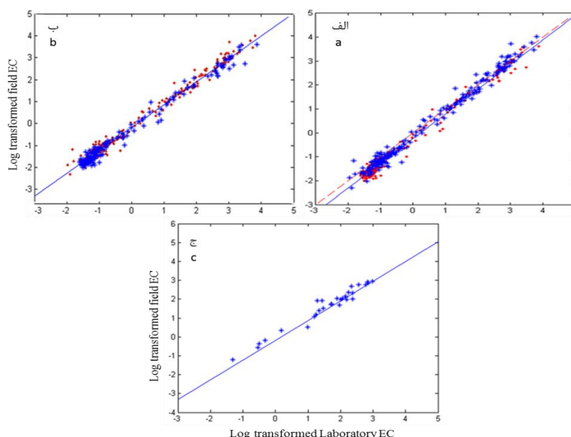
شکل ۳- واسنجی بین لگاریتم اندازه‌گیری‌های آزمایشگاهی (داده‌های مطمئن) و صحرایی (نامطمئن) هدایت الکتریکی خاک. الف) مدل خطی برازش شده بر روی سری اول و دوم داده‌ها به طور جداگانه؛ ب) مدل خطی برازش شده بر روی هر دو سری داده‌ها که کمترین مجموع مربعات خطای باقی‌مانده‌ها را به دست می‌دهد؛ ج) برازش مدل خطی محاسبه شده در قسمت ب، بر روی داده‌های صحرایی و آزمایشگاهی مربوط به سری پنجم نمونه‌برداری (پائیز ۱۳۹۳). در شکل الف و ب، رنگ آبی مربوط به پائیز ۱۳۸۸ و رنگ قرمز مربوط به بهار ۱۳۸۹ می‌باشد. Figure 3. Calibration between log transformed laboratory and field measurements of soil EC for a) the first and second sampling campaign; b) single line fitted on both first and second sampling campaigns; c) Calibration line from first two datasets fitted on 5th dataset (autumn 2014)
