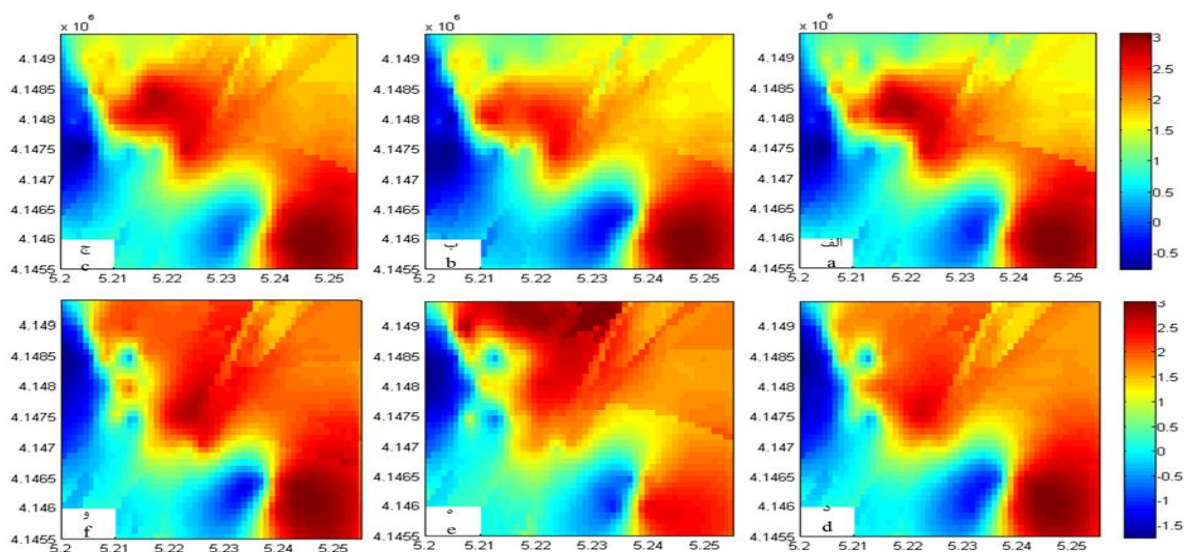
شکل ۶- تخمین مکانی- زمانی شوری خاک (درمقیاس لگاریتمی) با استفاده از روش انتروپی حداکثر اریب در منطقه مطالعاتی. الف تا و نشان‌گر سری چهارم الی نهم داده‌ها می‌باشند. الف) پائیز ۱۳۹۱؛ ب) پائیز ۱۳۹۳؛ ج) بهار ۱۳۹۴؛ د) پائیز ۱۳۹۴؛ ه) بهار ۱۳۹۵؛ و) پائیز ۱۳۹۵ Figure 6- Spatio-temporal prediction of soil salinity (on a log scale) using BME method at different time instants: a) autumn 2011, b) autumn 2014, c) spring 2015, d) autumn 2015, e) spring 2016, f) autumn 2016
